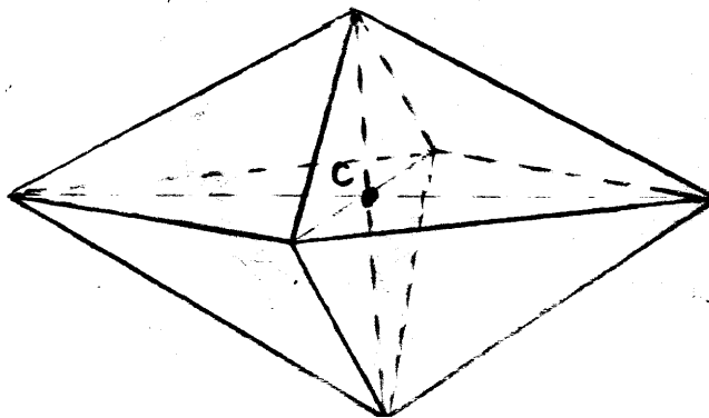
Рис. 5. Центрсимметрии - С
