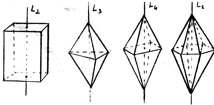
Рис. 3. Оси симметрии
