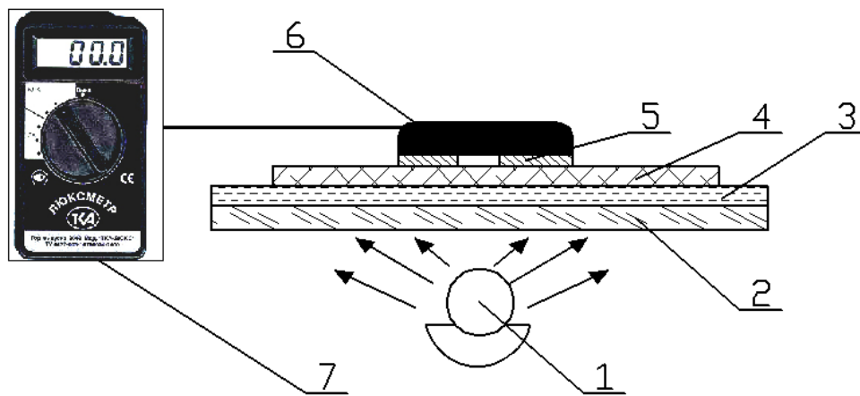
Рис. 1. Схема определения защитных свойств армирующего слоя композиционного слоистого материала с помощью люксметра: 1 – источник света; 2 – стекло; 3 – калька; 4 – рентгенограмма образцов; 5 – окно; 6 – датчик; 7 – люксметр
