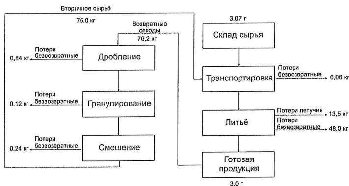
Схема материального потока производства детали из полипропилена методом литья под давлением
