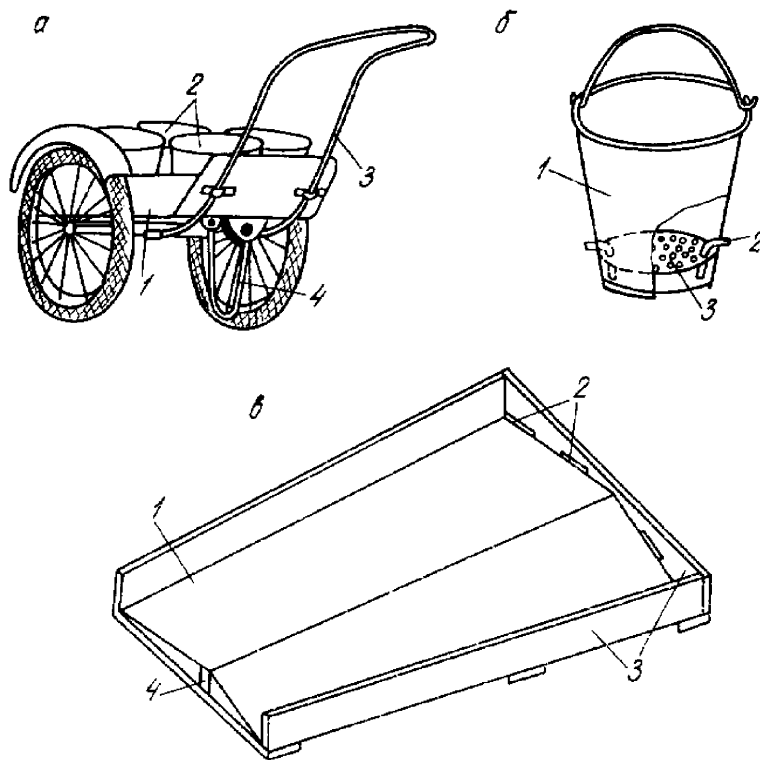
Рис. 53. Оборудование для сбора живицы: а - тележка для сбора живицы: 1 - кузов; 2 - ведра; 3 - ручки; 4 - упор; б - ведро для сбора живицы: 1 - десятилитровое ведро; 2 - патрубков-водослив; 3 - ложное дно; в - водосливная доска: 1 - водоотделяющая площадь; 2 - отверстия для слива воды; 3 - борта; 4 - брусок
