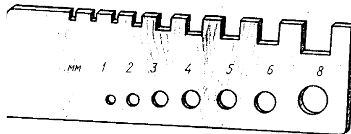
Рис. 67. Шаблон для измерения диаметра прутьев (в мм) с прямоугольными вырезами для неочищенного прута и отверстиями для прута чищенного
