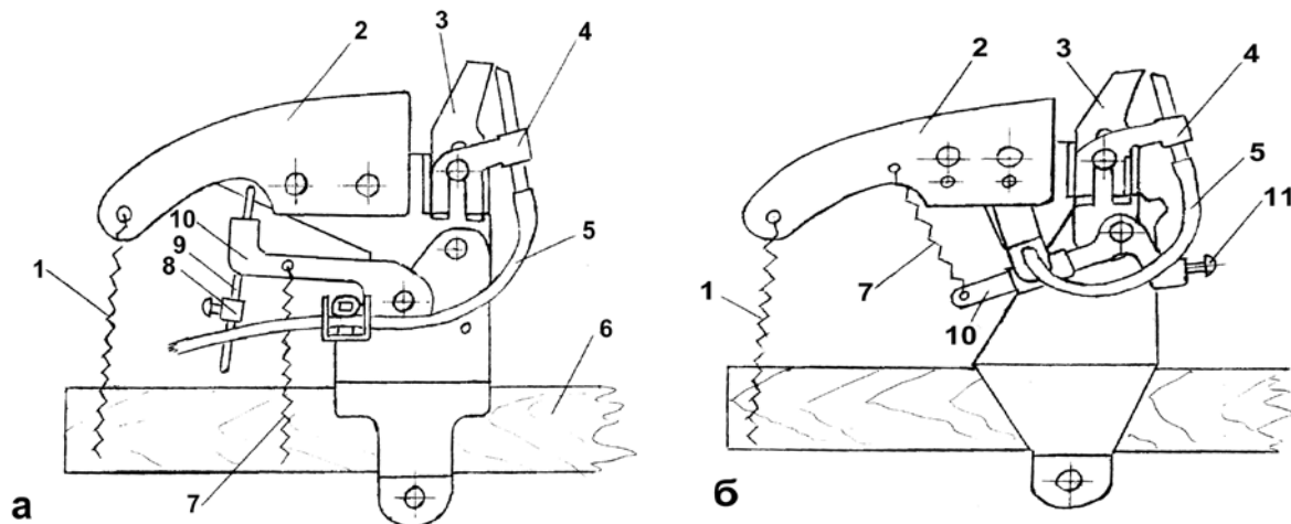
Рис. 48. Пневмохаки для подсочки с неагрессивными стимуляторами: а - химхак ЗН; б - химхак ЗНМ: 1 - возвратная пружина; 2 - регулятор; 3 - резец; 4 - дозатор; 5 - резиновая трубка; 6 - деревянная ручка; 7 - пружина пережимного устройства; 8 - стопор; 9 - тяга; 10 - рычаг; 11 - регулировочный винт
