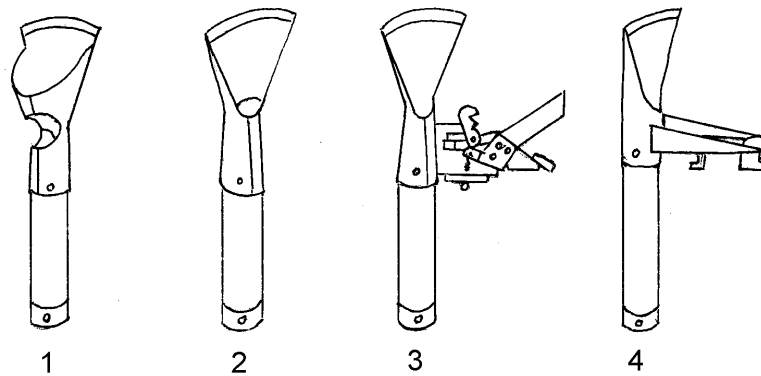
Рис. 32. Инструменты для изготовления щапа и установки приемников: 1 - стамеска Вольхина; 2 - стамеска Сидоровского; 3 - стамеска 2КМ; 4 - стамеска 2ПП
