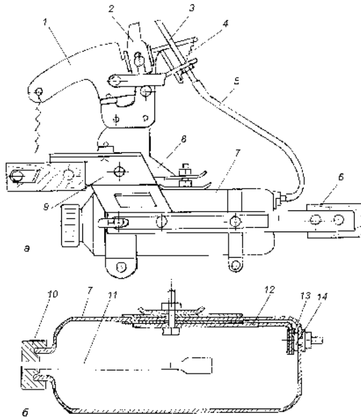
Рис. 42. Химхак 1Т:
