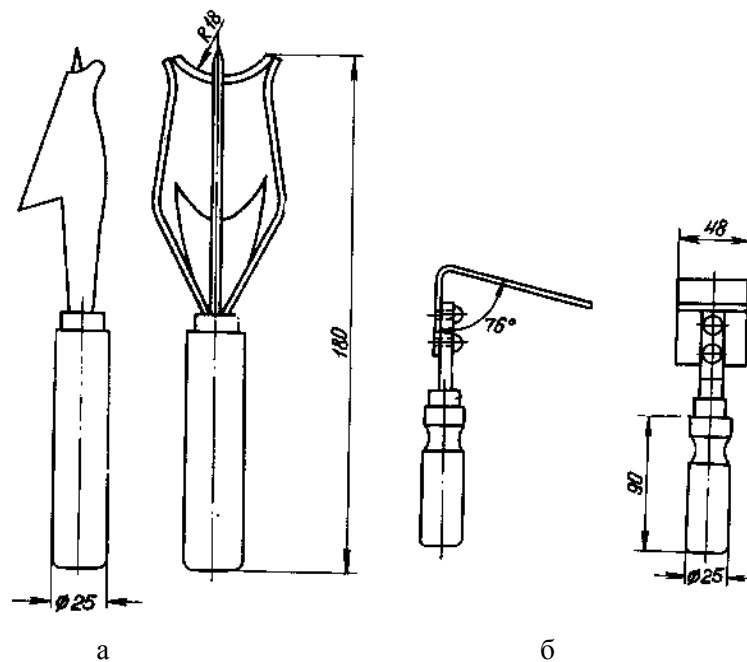
Рис. 17. Инструменты для сбора живицы при бесприемниковой подсочке: а - вскрыватель; б - выжиматель живицы
