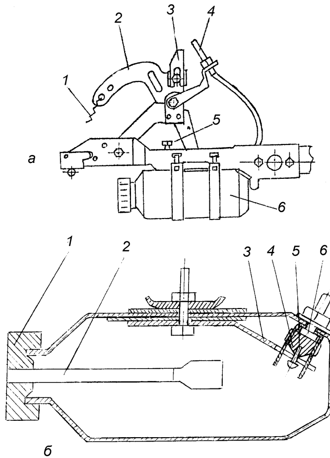
Рис. 43. Химхак 4ТМ:
