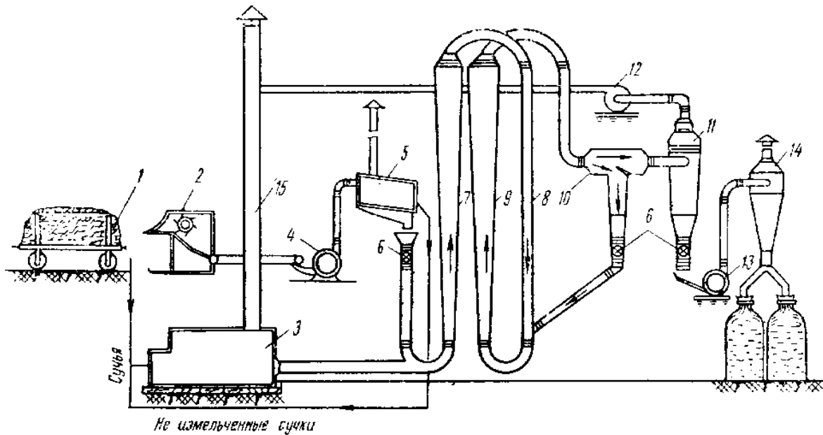
Рис. 86. Технологическая схема получения хвойной витаминной муки: 1 - вагонетка; 2 - хвоеотделитель; 3 - топка; 4 - дробилка; 5 - сито; 6 - дозатор; 7, 8, 9 - колонны; 10 - отделитель недосушенного продукта; 11 - циклон; 12 - вентилятор; 13 - дробилка для размола сухой хвой в муку; 14 - циклон для готовой муки; 15 - дымовая труба
