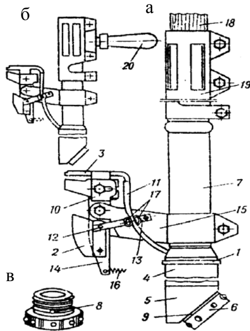
Рис. 46. Хак «Красноярец»:
