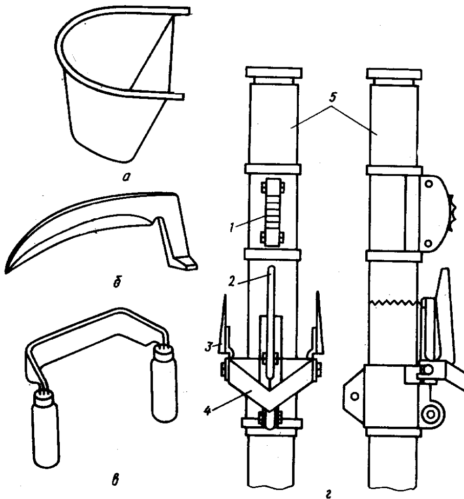
Рис. 55. Инструменты, используемые при осмолподсочке: а - хребтюг; б - косарь; в - двуручный скобель; г - химхак Ц-2: 1 - колесиковый дозатор; 2 - центральный регулятор; 3 - боковые регуляторы; 4 - резец; 5 - резервуар
