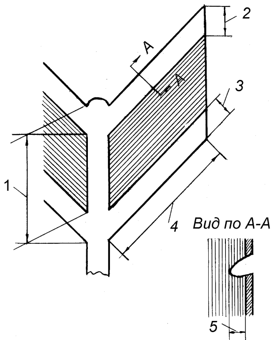
Рис. 12. Элементы карроподновки на ребристой карре: 1 - шаг подновки; 2 - высота подновки; 3 - ширина подновки; 4 - длина подновки; 5 - глубина подновки
