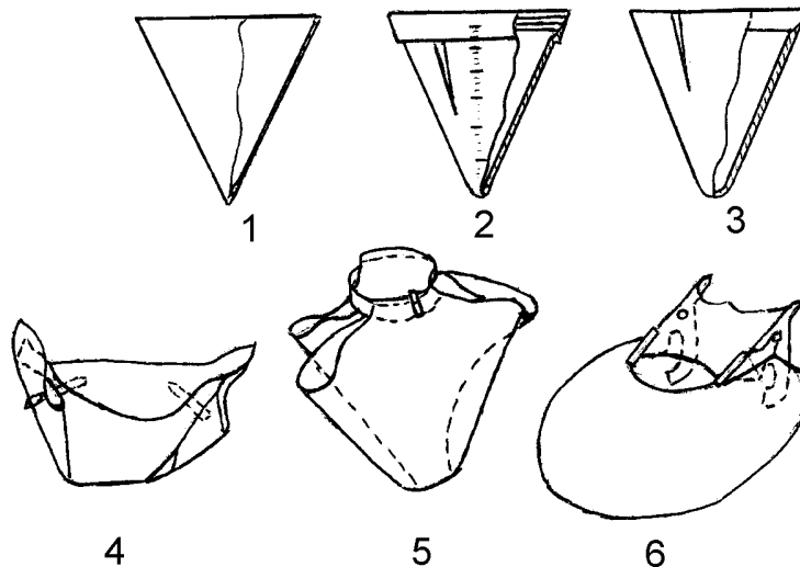
Рис. 33. Оборудование для подготовки карр: 1 - металлический конический приемник 1ПА; 2 - полиэтиленовый конический приемник 2ПА; 3 - полиэтиленовый конический приемник Борисовского завода; 4 - пленочный разворачивающийся приемник; 5 - пленочный приемник на манжете; 6 - крампон-держатель с крышкой
