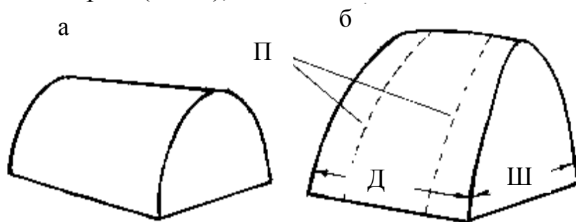
Рис. 114. Форма скирд:
