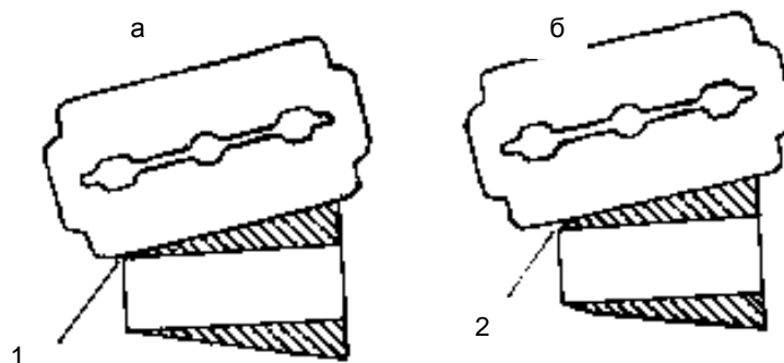
Рис. 37. Проверка правильности точки резца с помощью бритвенного лезвия: а - правильная, просвета (1) нет; б - неправильная, просвет (2) есть
