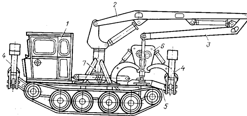
Рис. 60. Агрегат АКП-1:
