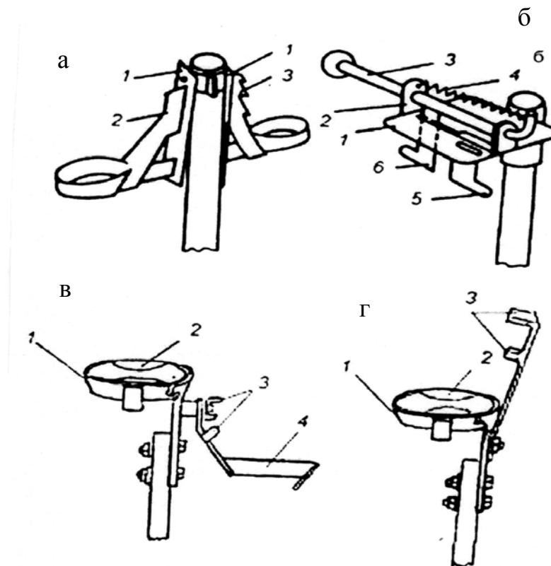
Рис. 50. Съемники живицеприемников:
