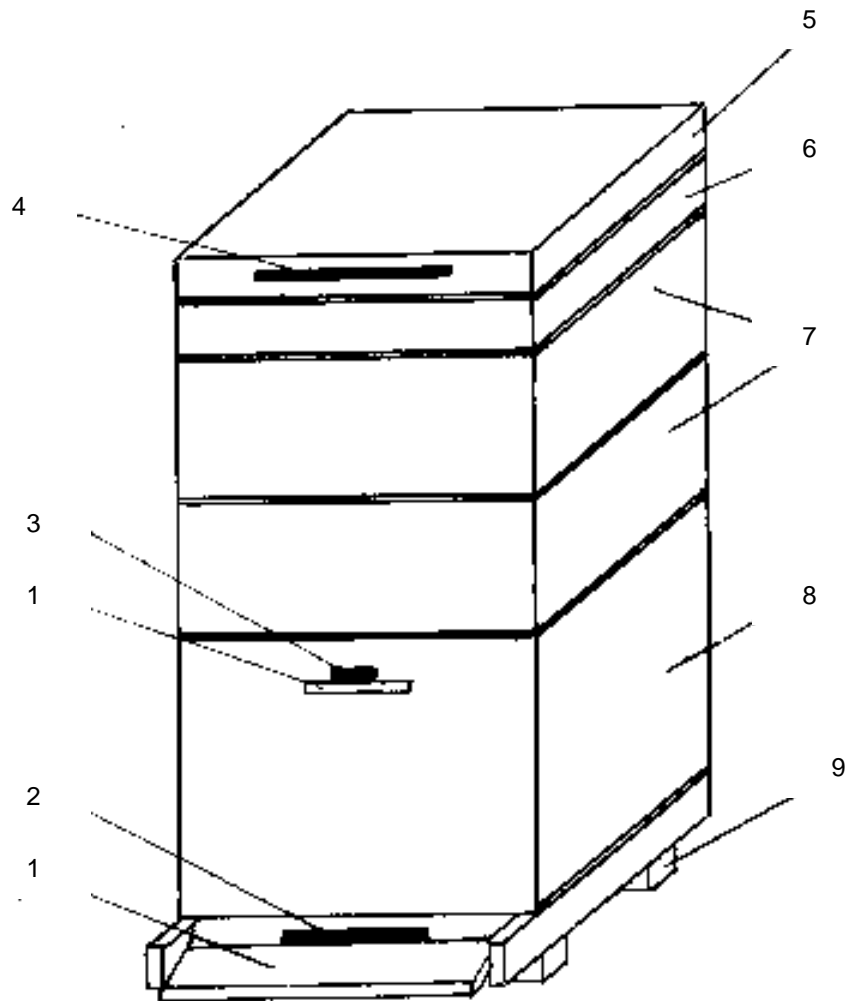
Рис. 115. Двенадцатирамочный однокорпусный улей с двумя магазинными надставками: 1 – прилетная дощечка; 2 – нижний леток; 3 – верхний леток; 4 – продух; 5 – крышка; 6 – подкрышник; 7 – магазинные надставки; 8 – корпус; 9 – подставка
