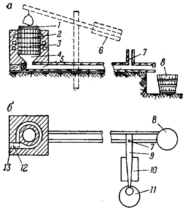
Рис. 81. Схема расположения оборудования вятского котла: а - разрез; б - план; 1 - крышка котла; 2 - котел; 3 - решетчатая корзина; 4 - выходное отверстие; 5 - канал; 6 - подъемник; 7 - стояк; 8 - приемник; 9 - патрубок; 10 - холодильник; 11 - приемник скипидара; 12 - дымовая труба; 13 - топка
