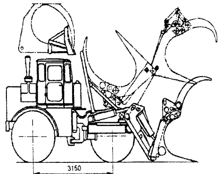
Рис. 3. Лесоштабелер ЛТ-163
