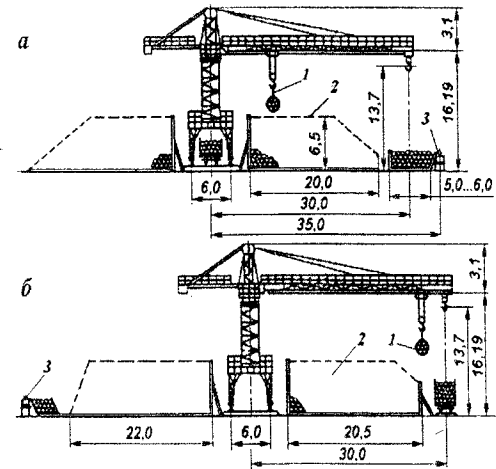
Рис. 2. Выгрузка бревен из подвижного состава башенным краном:
