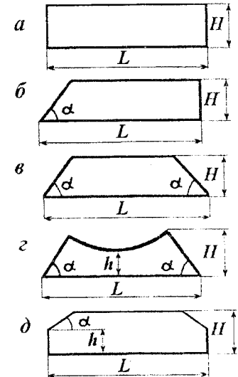
Рис. 4. Форма штабеля
