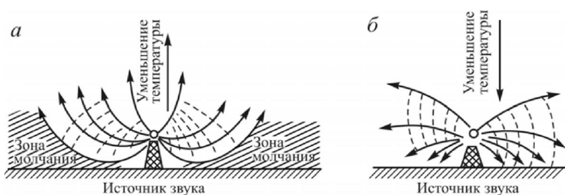
Рис. 1. Схематическая модель распространения акустической волны в зависимости от температуры: а – при увеличении (ночью); б – при снижении (днем)
