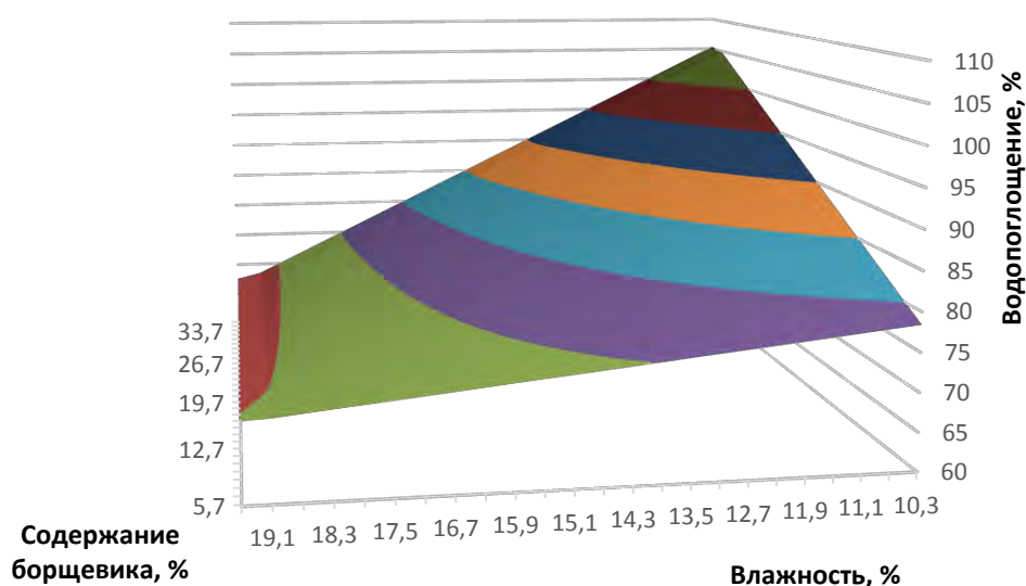
Поверхности зависимости твердости и водопоглощения РК-БС от содержания стеблей борщевика и ее фракционного состава
