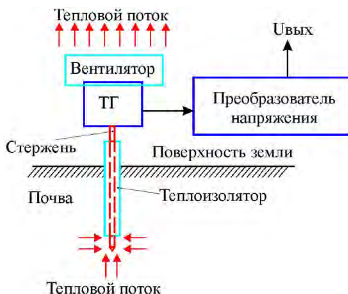
Рис. 2. Структурная схема альтернативного источника электропитания: ТГ – термогенератор
