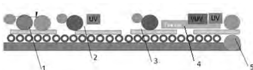
Рис. 2. Принципиальная схема линии лакирования «BARBERAN»: 1 – MENH; 2, 3 – BRB-2; 4 – НОК-14/2; 5 – CAL
