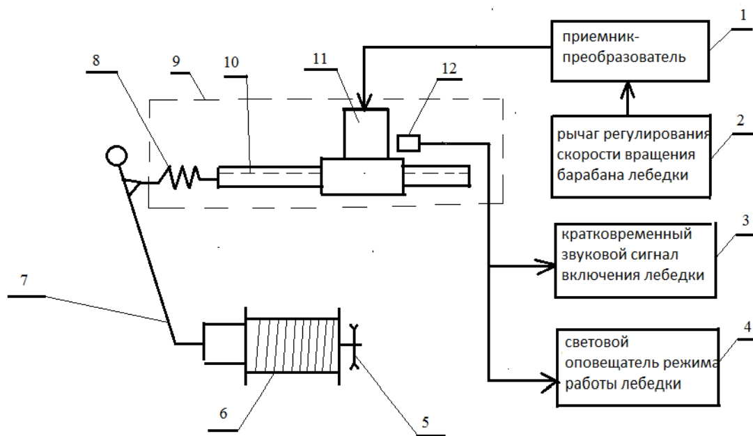
Рис. 2. Блок-схема МТР-1:
