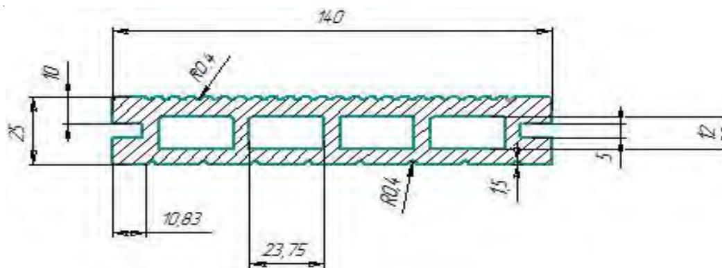
Сечение декинга
