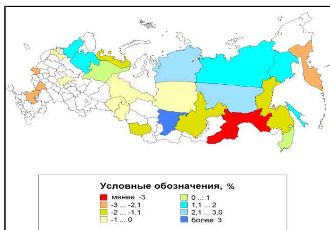
Изменение влажности воздуха в регионах РФ (1991-2018 гг.) по отношению к периоду (1961-1990 гг.)
