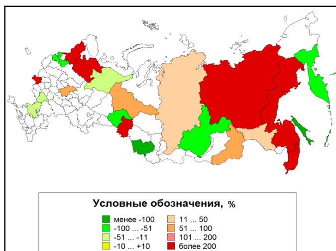
Изменение площади лесных пожаров в регионах РФ (2008-2018 гг.) по отношению к периоду (1991-2000 гг.)
