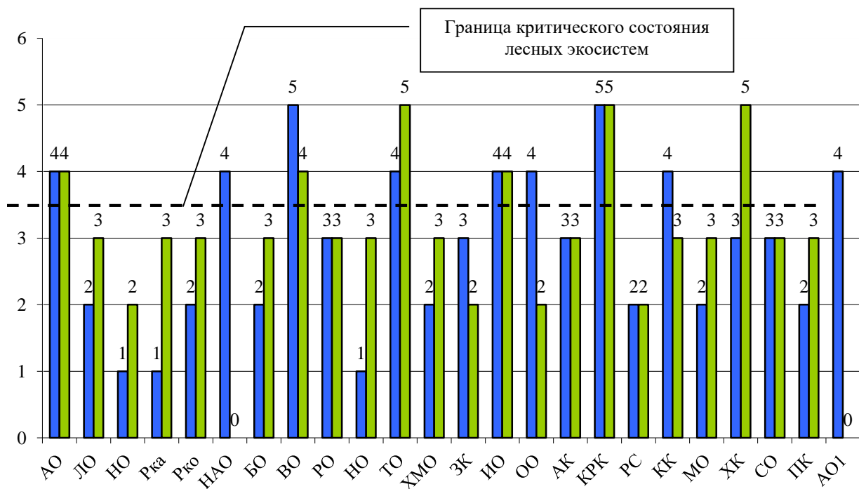
Рисунок 8 – Распределение региональных лесных экосистем по уровню индексов адаптационного потенциала (АО – Архангельская область; ЛО – Ленинградская область; НО – Новгородская область; Рка – Республика Карелия; Рко – Республика Коми; НАО – Ненецкий автономный округ; БО – Брянская область; ВО – Воронежская область; РО – Ростовская область; НО1 – Нижегородская область; ТО – Тюменская область; ХМО – Ханты-Мансийский автономный округ; ЗК – Забайкальский край; ИО – Иркутская область; ОО – Омская область; АК – Алтайский край; КРК – Красноярский край; РС – Республика Саха; КК – Камчатский край; МО – Магаданская область; ХК – Хабаровский край; СО – Сахалинская область; ПК – Приморский край; АО1 – Амурская область)
