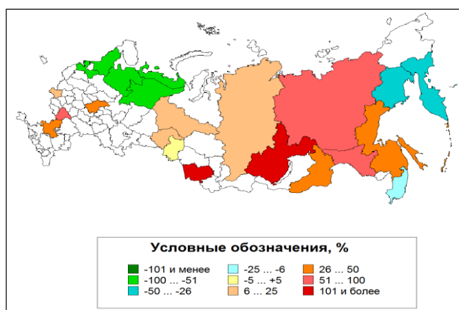
Изменение количества ОЯ в регионах РФ (2009-2018 гг.) по отношению к периоду (1991-2000 гг.)
