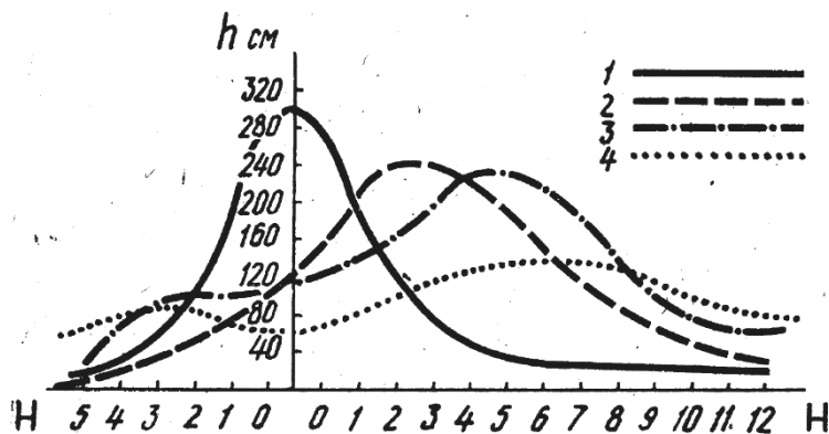
Рис. 17. Снеготложение ( h ) на полях, защищенных лесными полосами разной конструкции (по Трещевскому, Шаталову):
