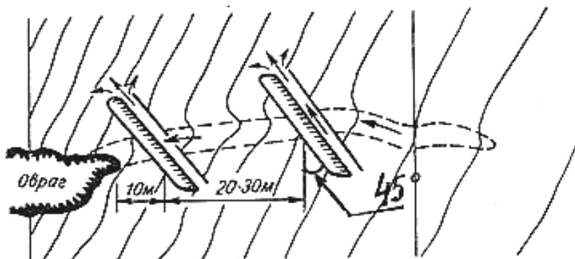
Рис. 8. Расположение распылителей стока на плане
