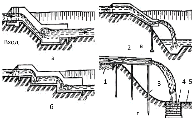
Рис. 10. Вершинные водосбросные сооружения: а – быстроток, б – перепад, в – консоль с наклонным лотком, г – консоль с прямым лотком; 1 – закрепленная вершина оврага, 2 – струнаправляющий лоток, 3 – опора лотка, 4 – водобойный колодец, 5 – укрепленная часть дна оврага
