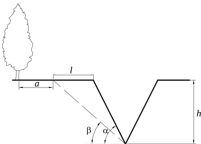
Рис. 7. Принцип расчета будущей бровки оврага
