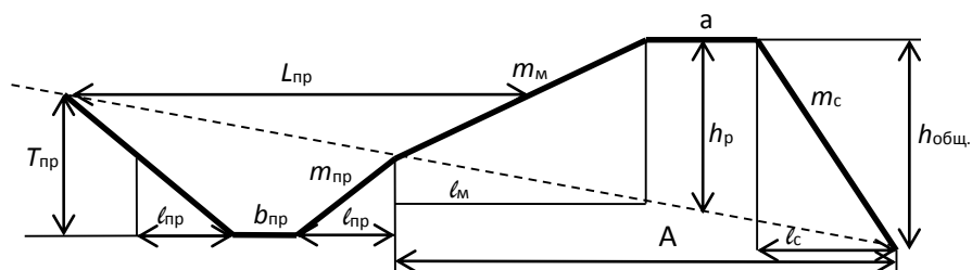
Рис. 13. Поперечное сечение водозадерживающего вала: A – ширина основания вала, a – ширина гребня вала, m_m – коэффициент мокрого откоса вала, i_m – заложение мокрого откоса вала, i_c – заложение сухого откоса вала, h_{\text{общ.}} – общая высота вала, h_p – рабочая высота вала, L_{\text{пр}} – длина прудка, b_{\text{пр}} – ширина основания прудка, T_{\text{пр}} – глубина прудка, i_{\text{пр}} – заложение откоса прудка, m_{\text{пр}} – коэффициент откоса прудка
