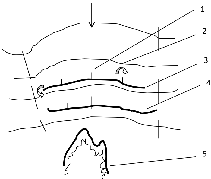
Рис. 12. Размещение водозадерживающих валов у вершины оврага: 1 – глухая перемычка; 2 – открытая перемычка; 3 – открытая «шпора»; 4 – глухая «шпора»; 5 – овраг
