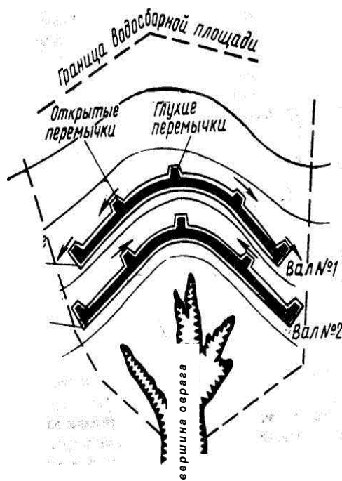
Рис. 9. Расположение водозадерживающего вала в вершине оврага
