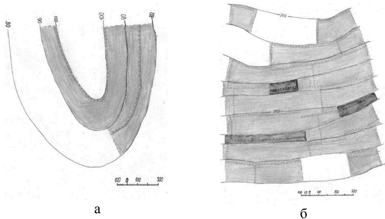
Рис. 14. Расположение водорегулирующих полос на водосборах рассеивающего типа: а – с равномерным падением склонов, б – с неравномерным падением склонов
