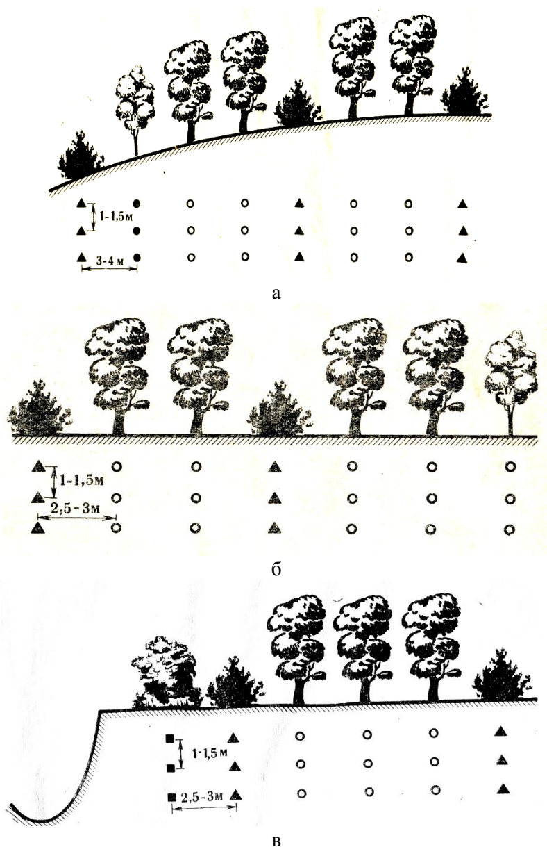
Рис. 19. Схемы размещения древесных и кустарниковых пород в защитных лесных полосах: а – прибалочная лесная полоса; б – водорегулирующая лесная полоса; в – приовражная лесная полоса
