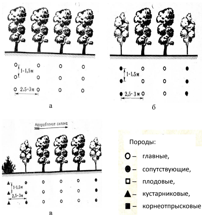
Рис. 18. Схемы размещения древесных и кустарниковых пород в защитных лесных полосах: а, б – в полезащитных лесных полосах; в – водорегулирующая лесная полоса
