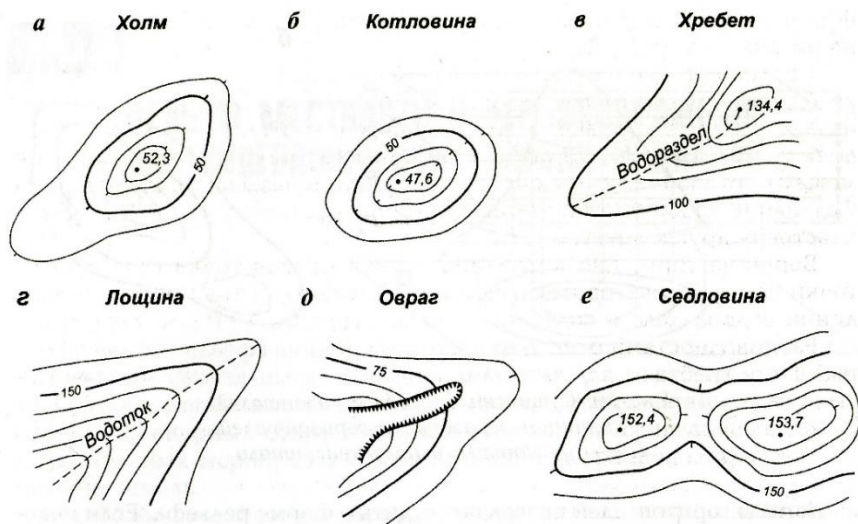
Рис. 1. Основные формы рельефа (по Покладу, Гридневу)
