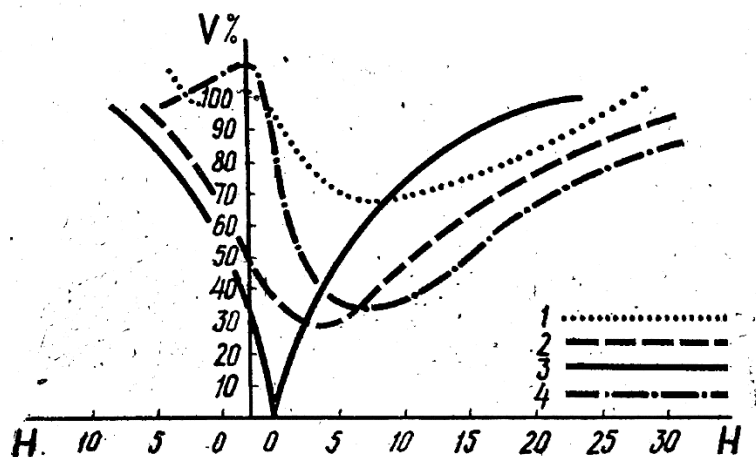
Рис. 16. Влияние лесных полос разной конструкции на скорость ветра (по Трещевскому, Шаталову):
