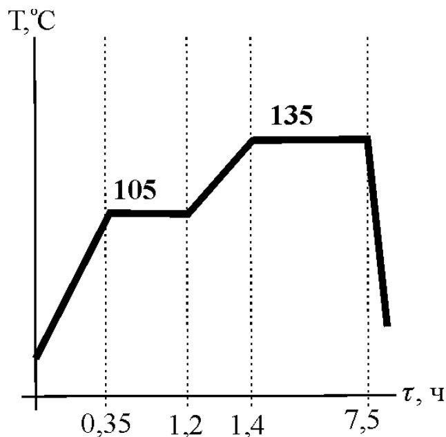
Рис. 1. График варки целлюлозы
