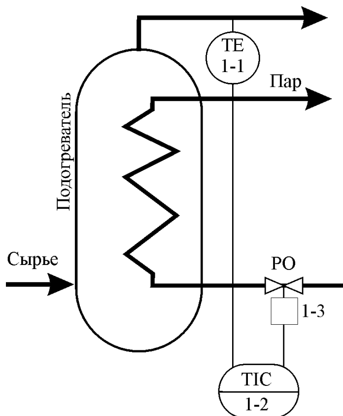
Рис. 2. Функциональная схема регулирования температуры в подогревателе
