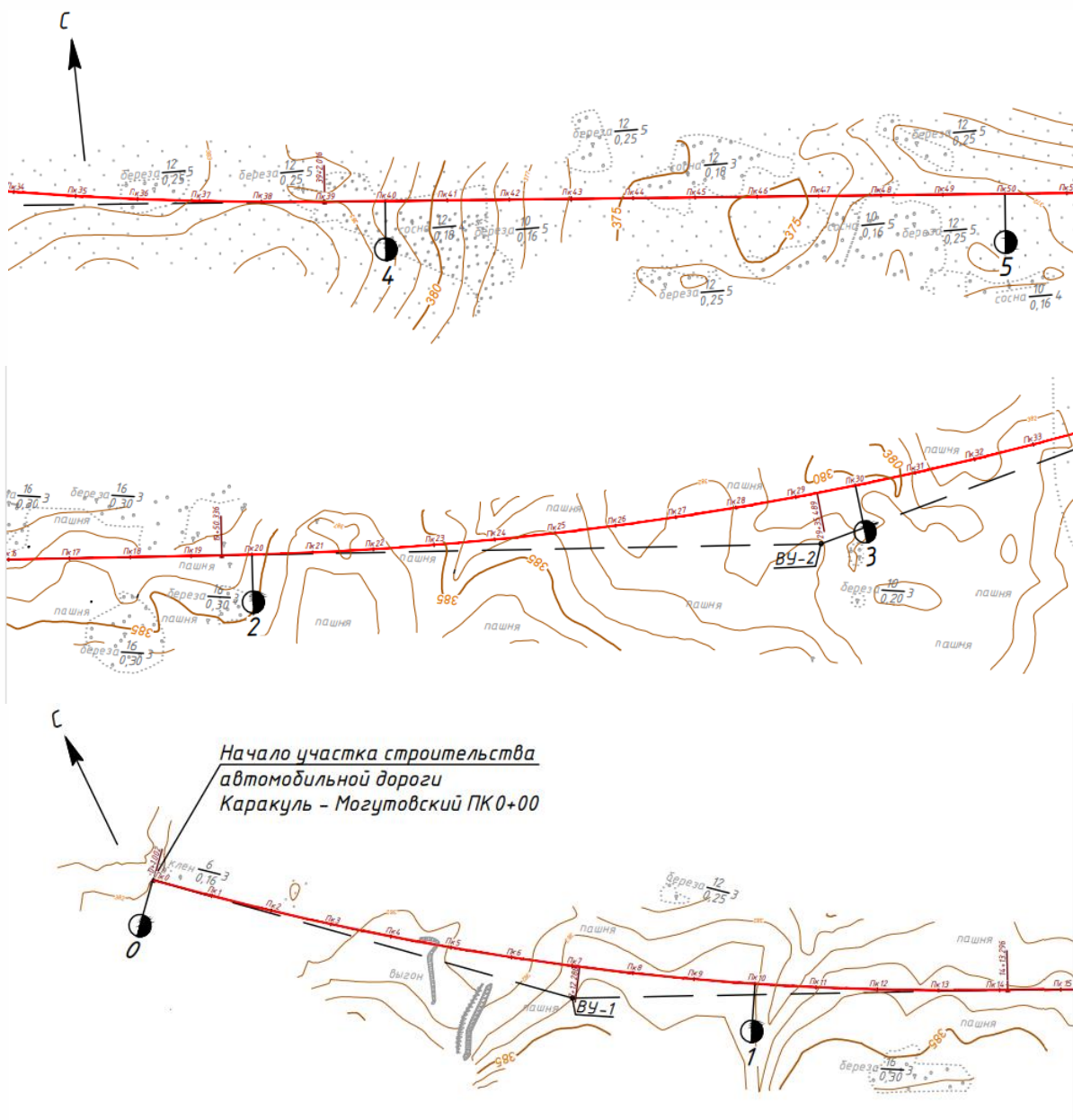
Рис. 2.8. План трассы
