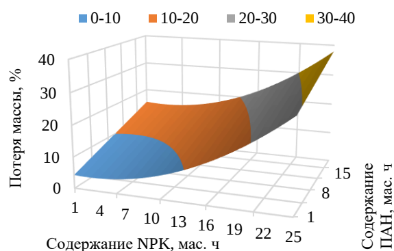
Рис. 10. Зависимость потери массы после выдержки в грунте в течение 60 суток от содержания NPK-удобрения и ПАН при содержании ДМ 20 мас. ч.
