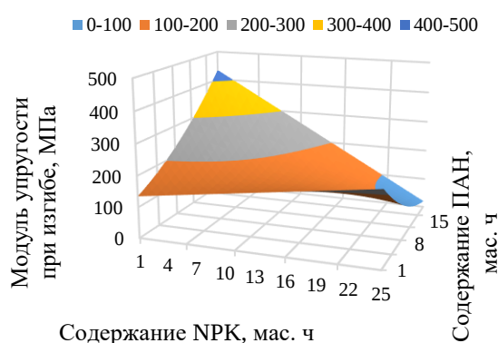
Рис. 23. Зависимость модуля упругости при изгибе от содержания NPK и ПАН при содержании ДМ 20 мас. ч.
