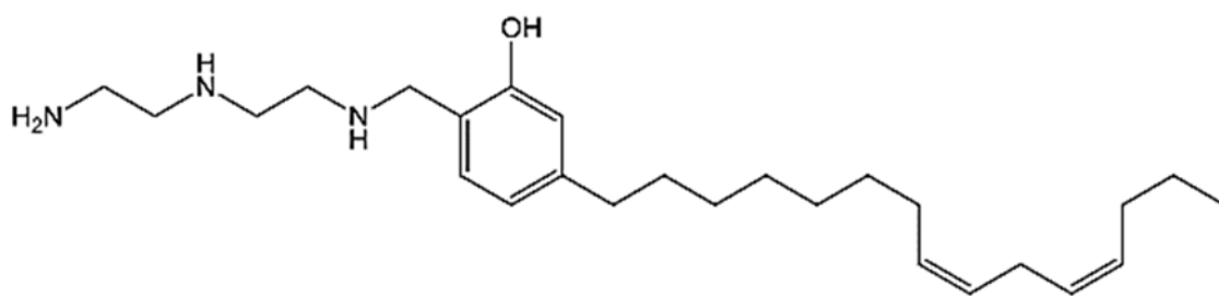
Рис. 1. Структурная формула Кардамина-Д [1]
