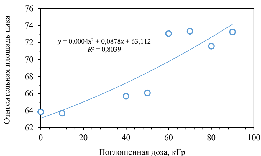
Рис. 2. Изменение относительной площади пика при 3488\text{ см}^{-1} в процессе радиолитического деацетилирования пленок из ацетата целлюлозы
