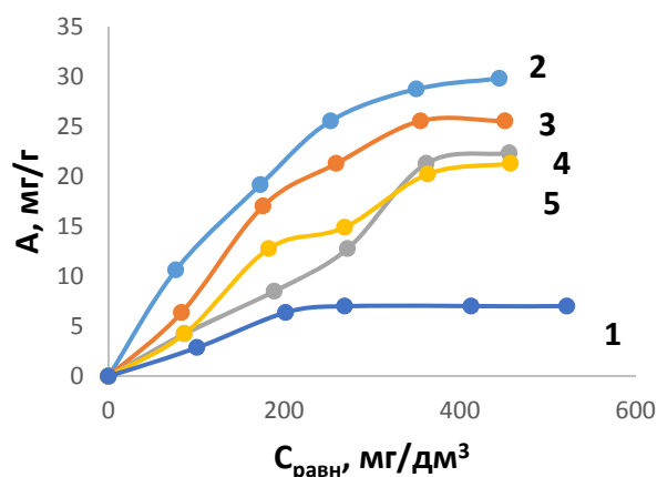
Изотермы сорбции ионов меди(II) сорбентами на основе опилок ясеня
