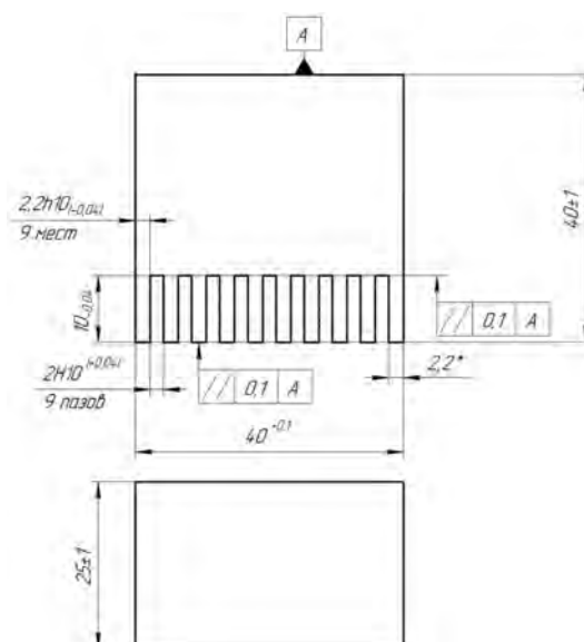
Рис. 1. Параметры применяемого инструмента – пуансона
