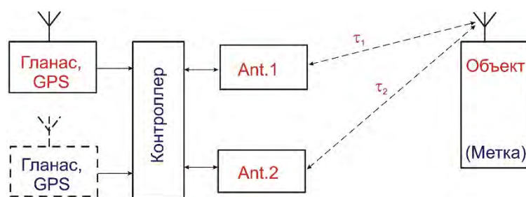
Рис. 1. Структурная схема поиска RFID-меток на участке леса
