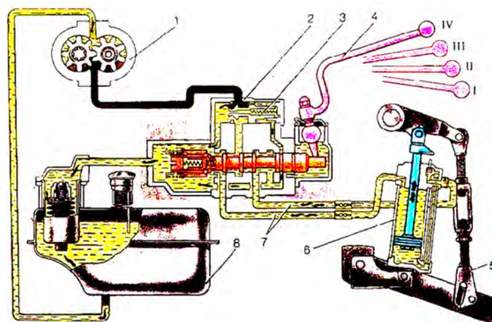
Рис. 1. Общий вид гидравлической системы привода навесного оборудования трактора МТЗ BELARUS 82: 1 – масляный насос; 2 – распределитель; 3 – перепускной клапан; 4 – рукоятка распределителя; 5 – механизм навески; 6 – силовой гидроцилиндр; 7 – маслопроводы; 8 – масляный бак; I – подъем; II – нейтральное; III – опускание принудительное; IV – плавающее
