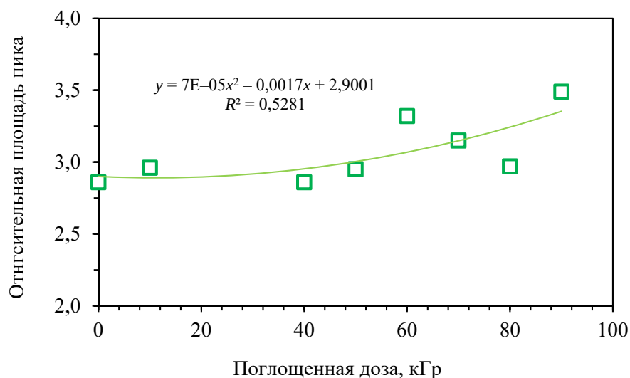
Рис. 3. Изменение относительной площади пика при 1744\text{ см}^{-1} в процессе радиолитического деацетилирования пленок из ацетата целлюлозы
