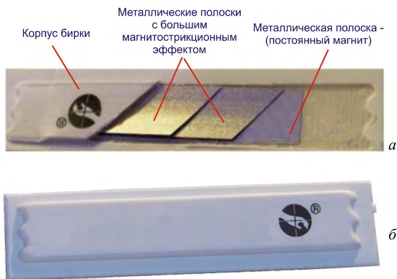
Рис. 2. Конструкция акустомангнитной (магнитострикционной) метки: а – вид в разрезе; б – вид общий
