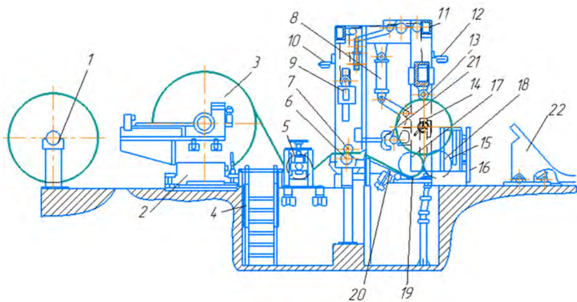
Рис. 1. Схема ПРС:
