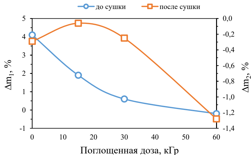
Рис. 3. Изменение массы образцов отвержденной Кардамино-Д эпоксидной смолы после экспонирования в 10%-ном растворе HCl
