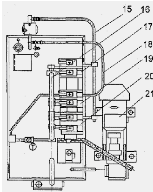
Рис. 8. Маслостанция. Вид сверху
