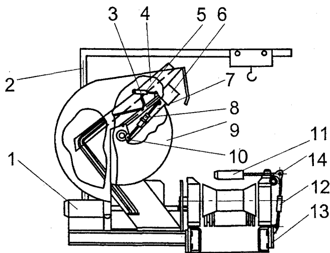
Рис. 4. Блок раскряжевки
