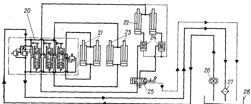
Рис. 11. Гидросистема валочно-пакетирующей машины ЛП-2: а – гидропривод, расположенный на поворотной платформе машины; б – гидропривод, расположенный на неповоротной части машины
