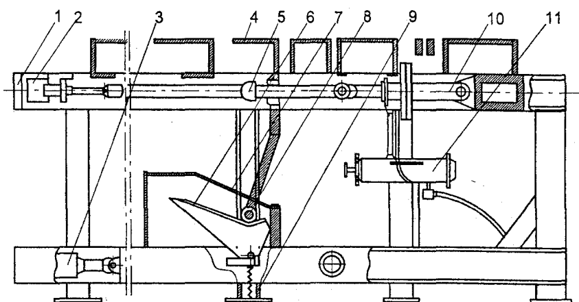
Рис. 5. Стол приемный
