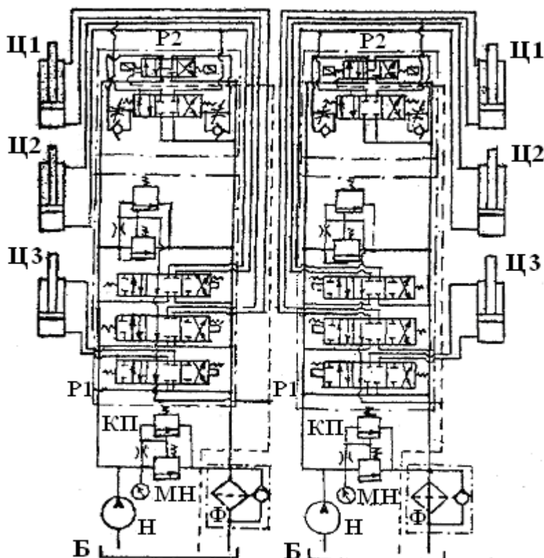
Рис. 3. Гидросистема манипулятора двухстрелового ЛО-13С:
