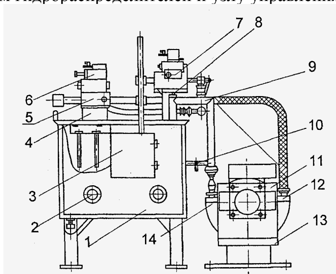
Рис. 7. Маслостанция. Вид сбоку
