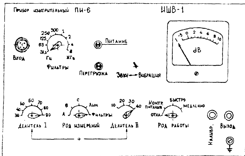
Рис. 2. Лицевая панель измерительного прибора ИШВ-1
