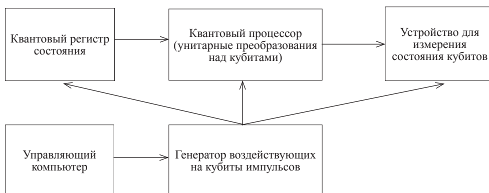
Рис. 2. Схематическая структура квантового компьютера (Пахомов, 2007)
