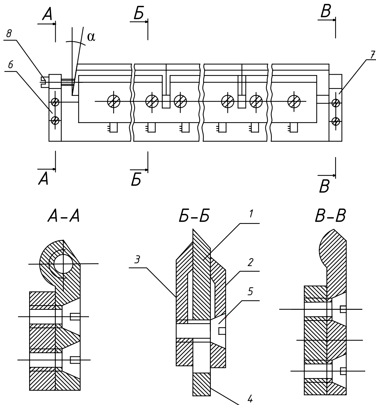
Рисунок 1 – Сборный нож
