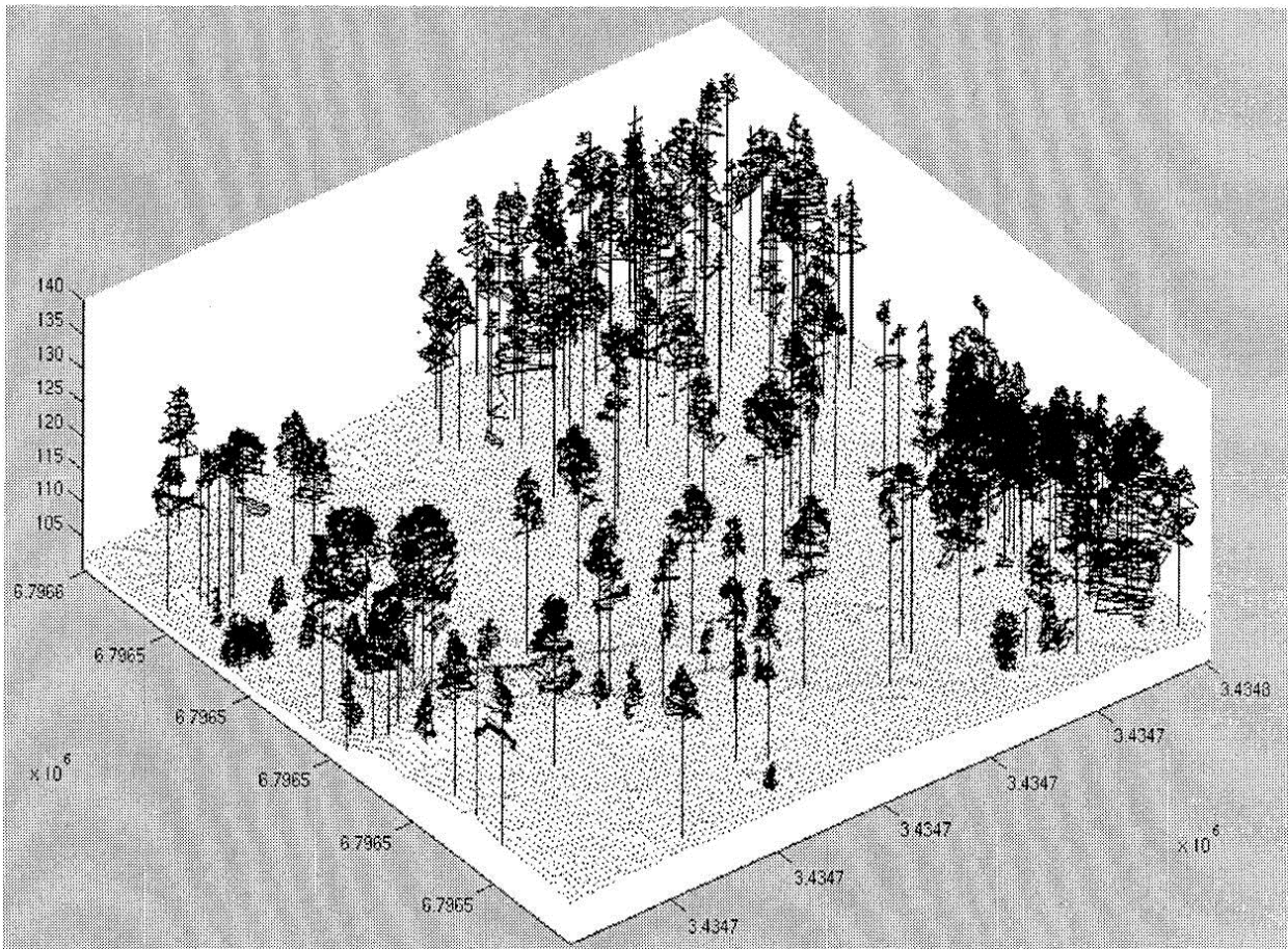
Рис. 4.15. Трехмерная (3-D) реконструкция морфоструктуры древостоя по данным лазерной локации. По результатам наземных обмеров крон 50 деревьев установлено, что множественное лазерное сканирование дает более точную картину профиля лесного полога, по крайней мере, верхней его части, по сравнению с наземной съемкой (Pyysalo, 2000)
