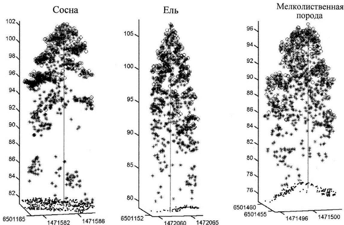
Рис. 4.2. Множественная регистрация бортовым носителем отраженных лазерных импульсов (laser points) формирует вертикальный профиль деревьев на примере трех древесных пород (Næsset et al., 2004)
