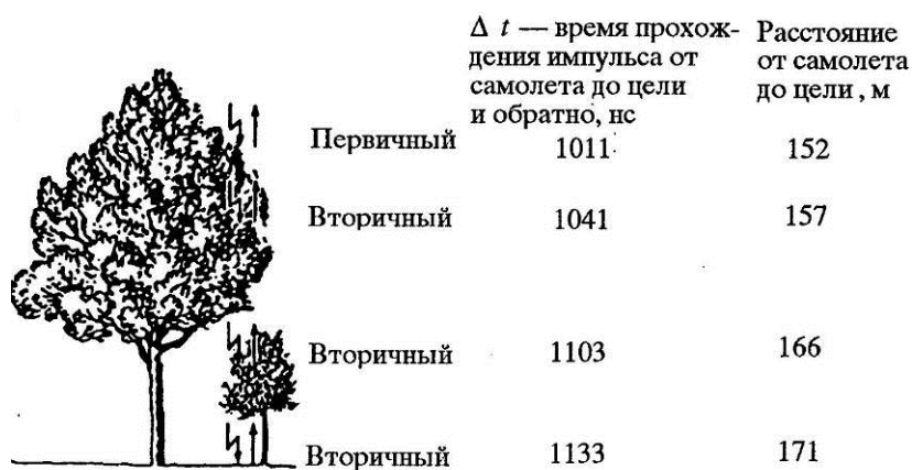
Рис. 4.3. Схема множественного отражения лазерного импульса от лесного полога высотой 18 м (Nelson et al., 1988).
