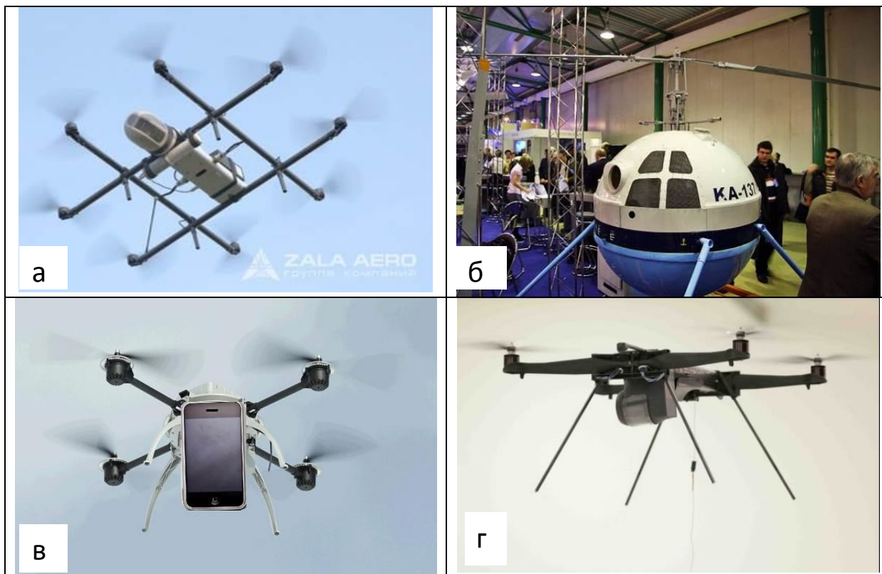
Рис. 4.8. Беспилотные вертолеты: (а) «ZALA 421-22», взлётная масса 8 кг ( http://zala.aero/category/production/bla/helicopters/ ); (б) Ka-137. Многоцелевой беспилотник, взлетная масса 280 кг ( http://www.helicopter.su/enc/vertoleti/ka-137.html ); (в) «летающий смартфон» ( http://www.popsci.com/category/tags/uas ); (г) дрон PARC на силовом кабеле длиной 300 м с системой камер высокого разрешения ( http://paranormal-news.ru/news/letajushhij_robot_shpion_sposoben_ostavatsja_v_vozduke_vechno/2012-12-06-5788 )
