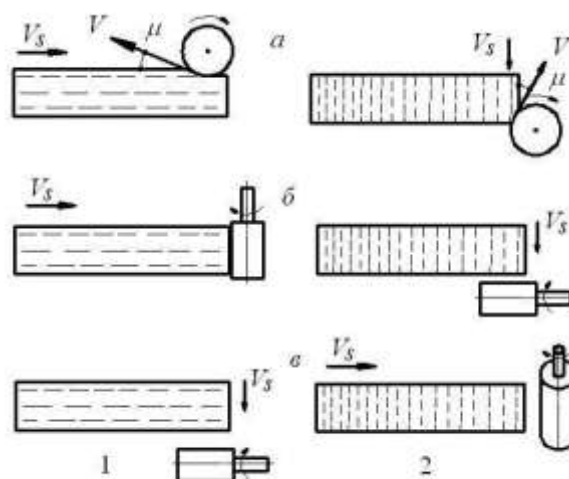
Рис. 1. Виды фрезерования древесностружечных плит плоского 1 и экструзионного 2 прессования:
