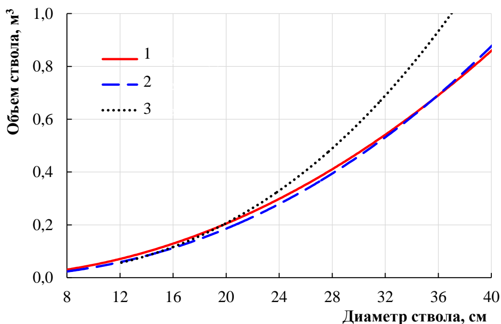
Рис. 5.5. Кривые объемов учетных деревьев березы повислой, построенные по данным разработанных таблиц объемов (1), ПИК (2) и таблиц Л.А. Лысова (3)
