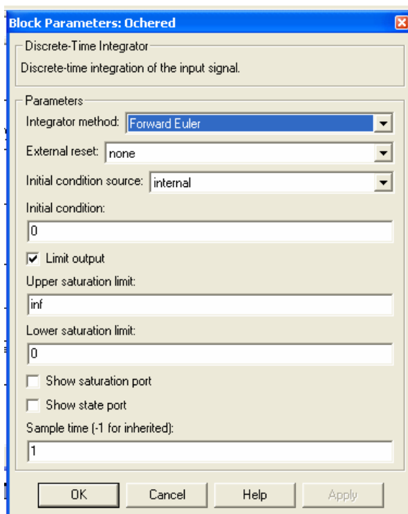
Рис. 3.2. Настройка блока Discrete-TimeIntegrator .
