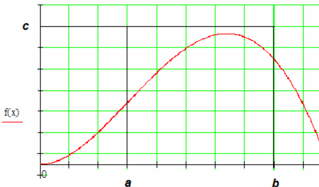
Рис. 2.12. Пример кривой, интеграл которой надо посчитать
