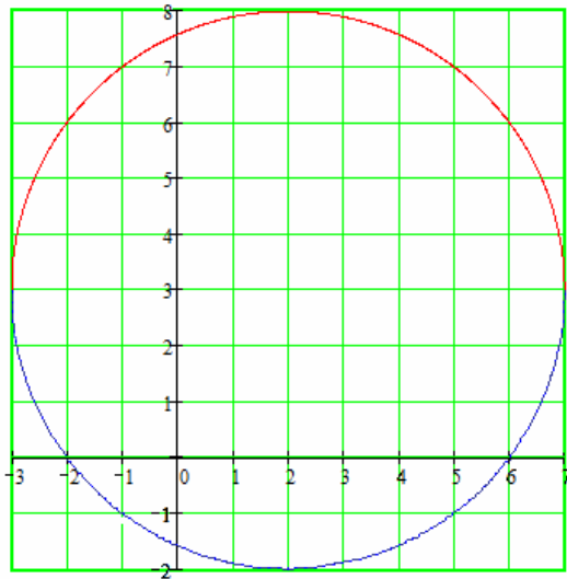
Рис. 2.1. Круг, вписанный в квадрат
