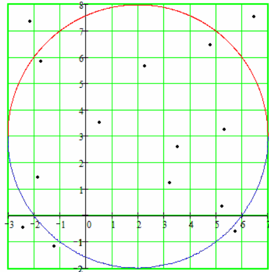
Рис. 2.2. Точки, случайно разбросанные по квадрату
