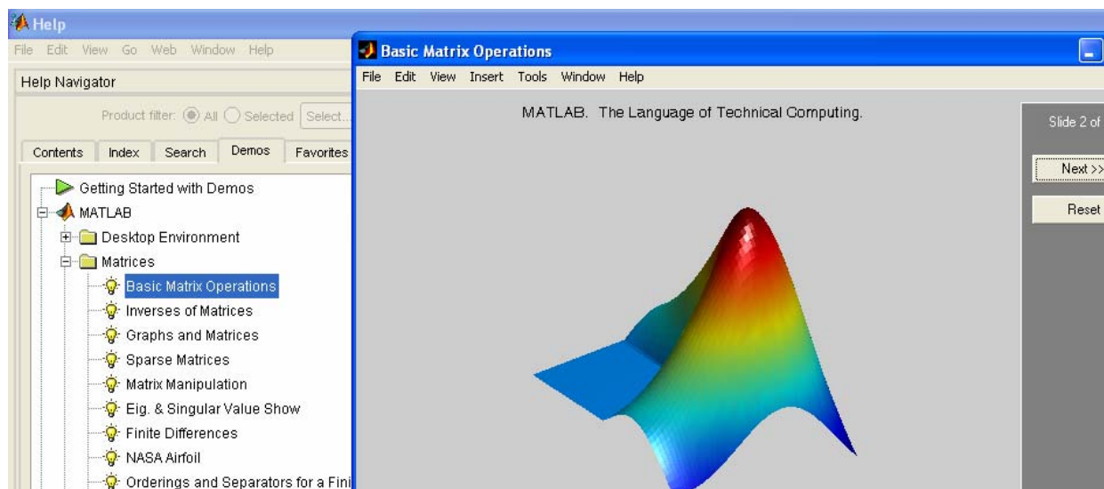
Рис.1.5. Демонстрация основных матричных операторов
